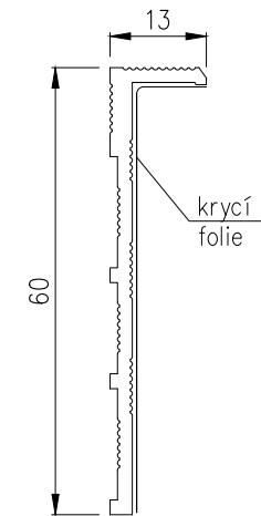
soklová lišta LINUS 13
