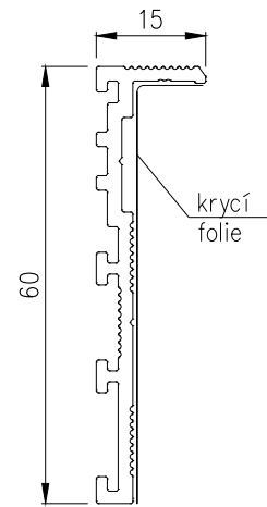
soklová lišta LINUS 15
